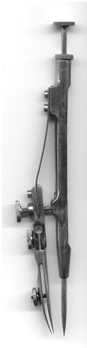
Циркуль с рейсфедером для построения окружностей малого диаметра («балеринка»)
